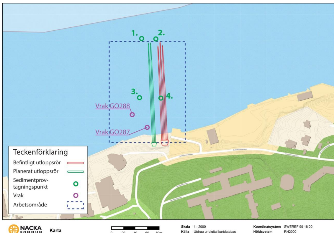
Figur 11. Planerat arbetsområde, punkter för sedimentprovtagning samt lägen för möjliga fartygslämningar.
