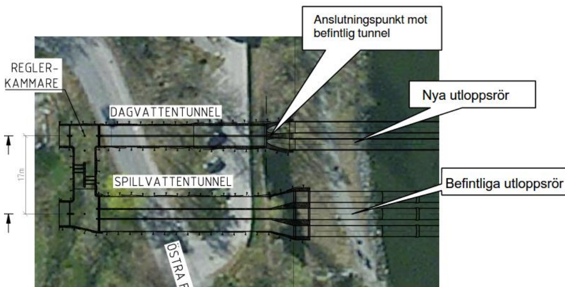
Figur 5. Bilden visar befintlig reglerkammare, dagvattentunnel, spillvattentunnel och utloppsror. De nya utloppsrören ansluts mot befintlig dagvattentunnel. Källa: SFAR Henriksdals utlopp Förstudie.
