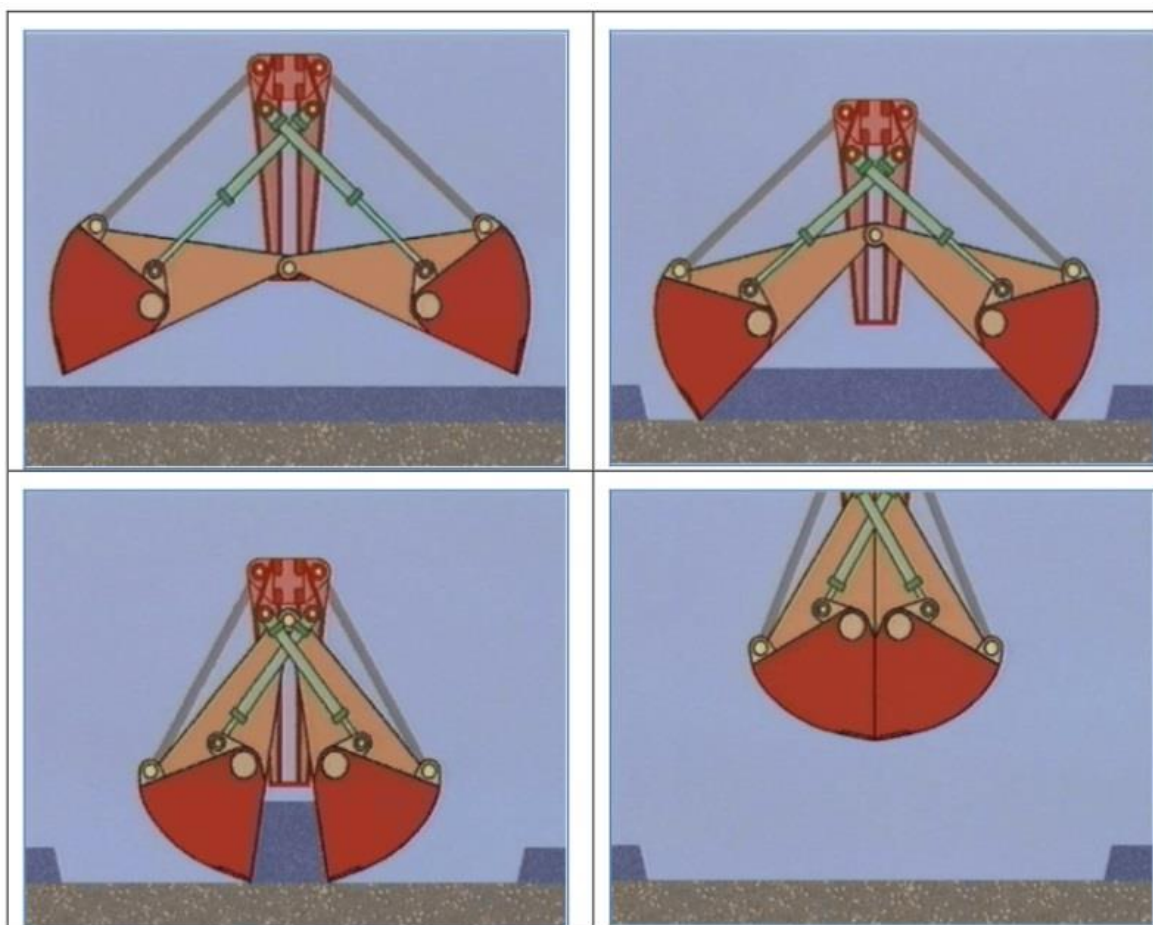
Figur 6. Illustration av miljöskopa. Källa: Teknisk beskrivning Grundläggning av utloppsledningar, Henriksdalsverket.
