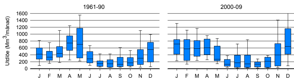
Figur 4. Fördelningen av Mälarens utflöde under året, perioderna 1961-1990 och 2000-2009.
