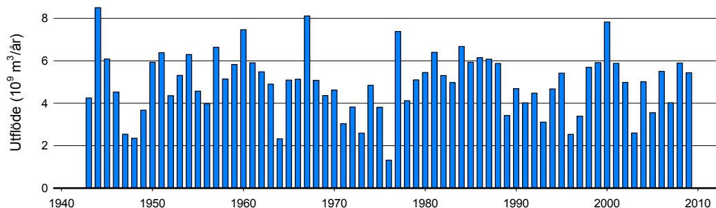
Figur 3. Mälarens utflöde 1943–2008, miljarder kubikmeter (kubikkilometer) per år.
