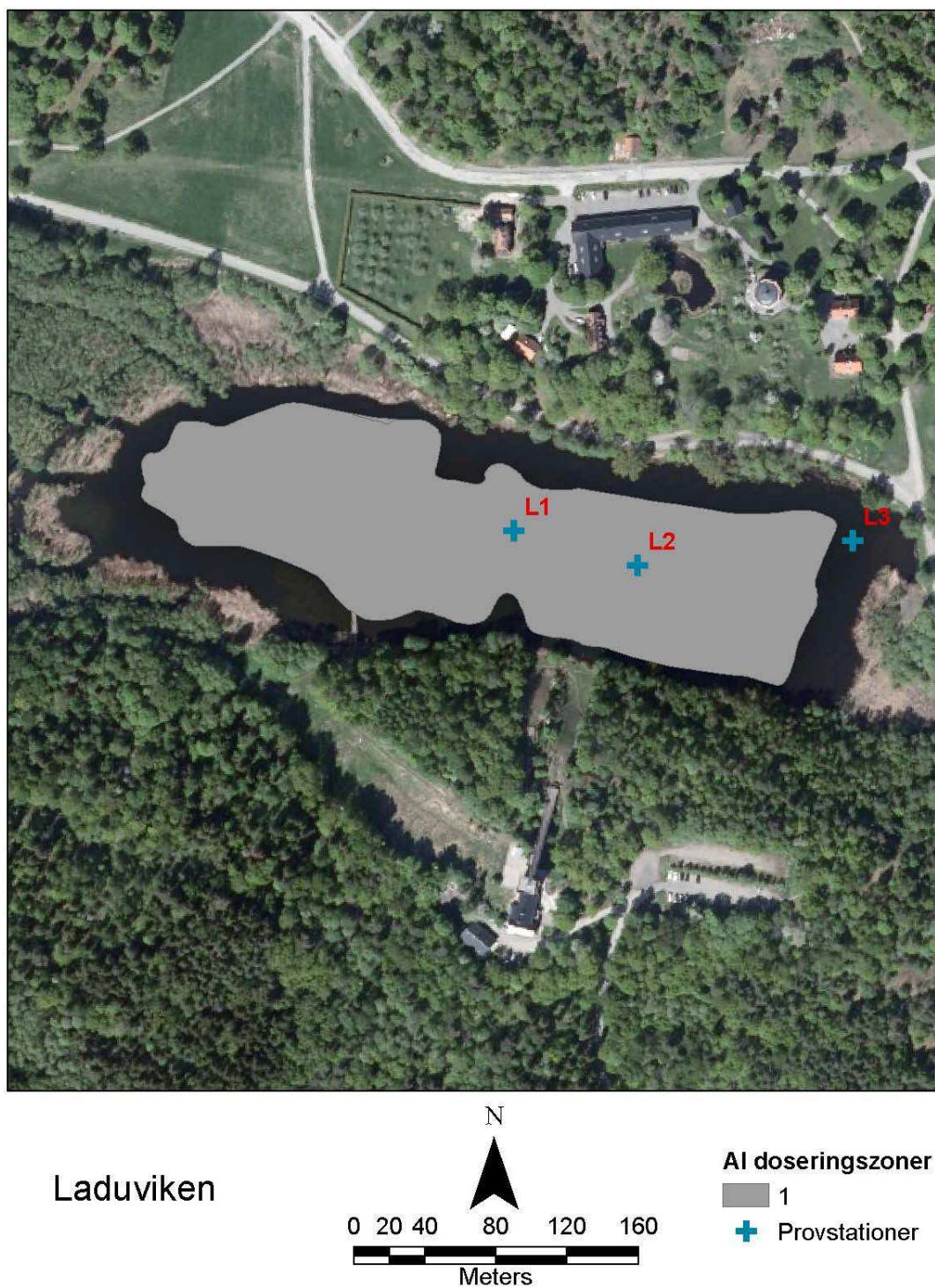
Figur 19. Behandlingszoner för aluminium i Laduviken.
