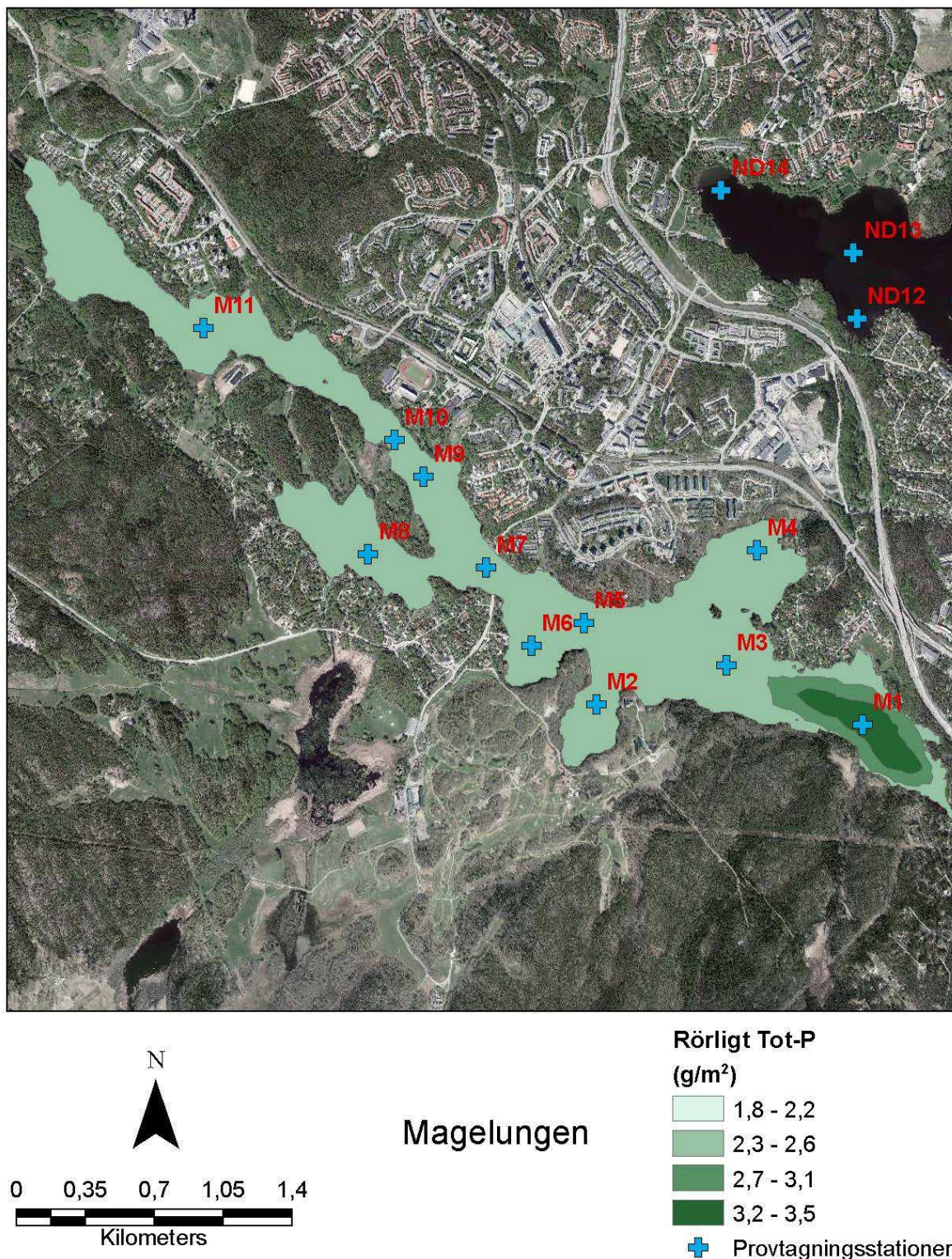
Figur 9. Rörliga fosforformer (mobilt och organiskt P) i sediment i Magelungen Kors visar där sediment provtogs i november 2016.
