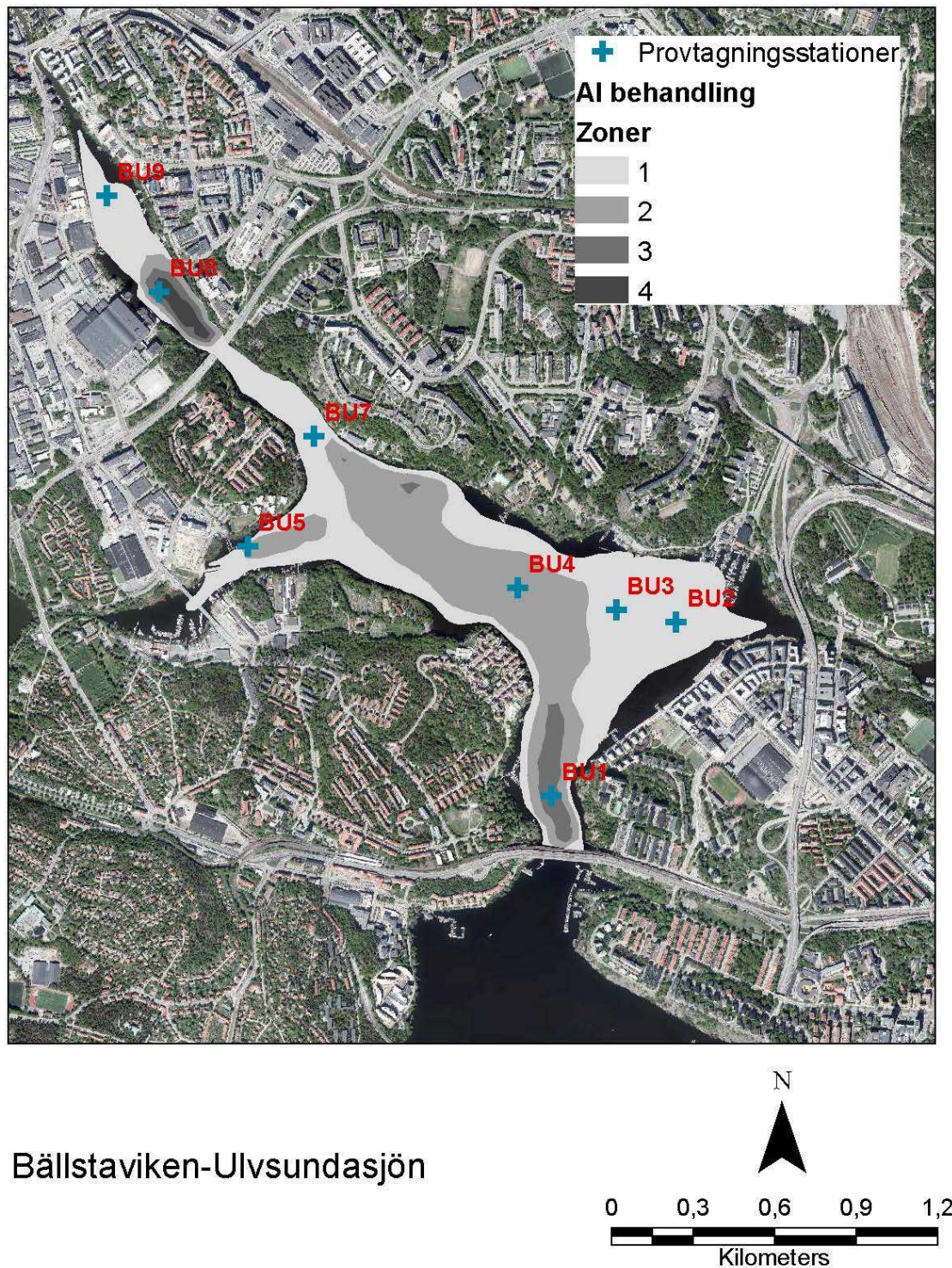
Figur 20. Behandlingszoner för aluminium i Bällstaviken-Ulvsundasjön.
