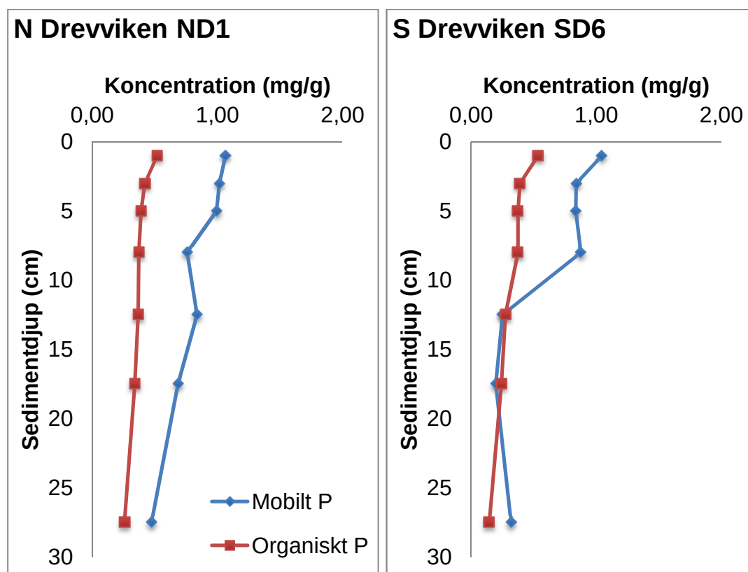
Figur 2. Mobila och organiska fosforkoncentrationer i Drevvikens sediment (proppar ND1 och SD6)
