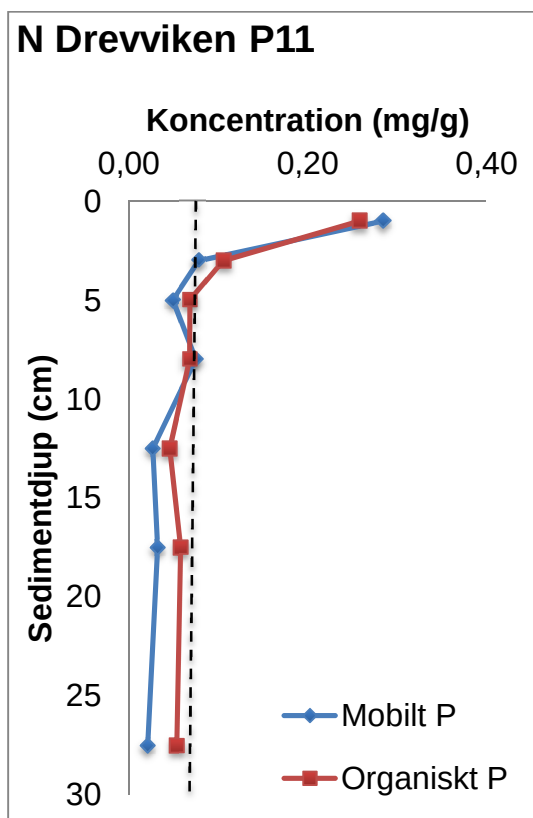
Figur 1. Mobil och organisk fosfor i propp 11 från Drevviken. Bakgrundskoncentration för organisk P visas med streckade linjen.
