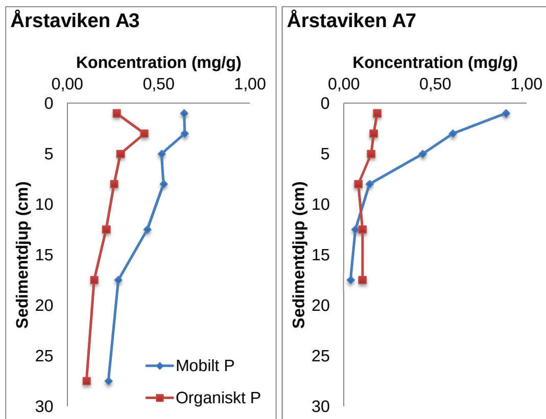
Figur 4. Koncentrationer av mobil och organisk fosfor i grundare (A7) och djupare (A3) delar av Årstaviken. Bara 20 cm sediment kunde hämtas i grundare delar där sedimentpropp A7 togs.
