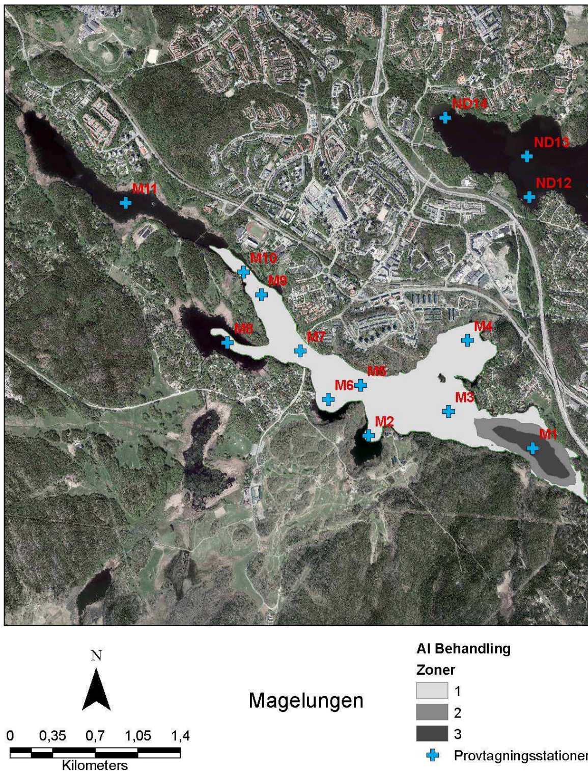
Figur 18. Behandlingszoner för aluminium i Magelungen.
