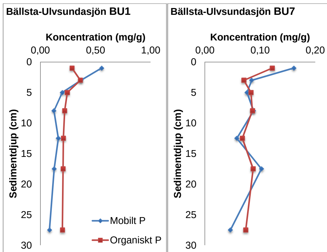
Figur 11. Koncentrationer av mobil och organisk fosfor i grundare (propp BU7) och djupare delar (propp BU1) av Bällstaviken-Ulvsundasjön.
