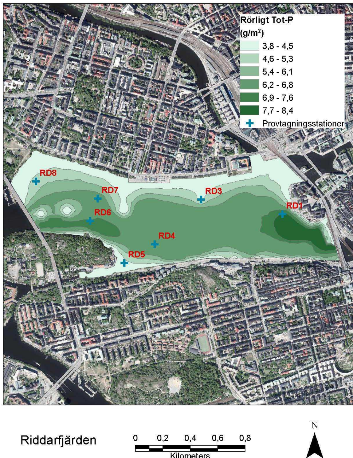
Figur 7. Rörliga fosforformer (mobilt och organiskt P) i sediment i Riddarfjärden. Kors visar där sediment provtogs i november 2016.
