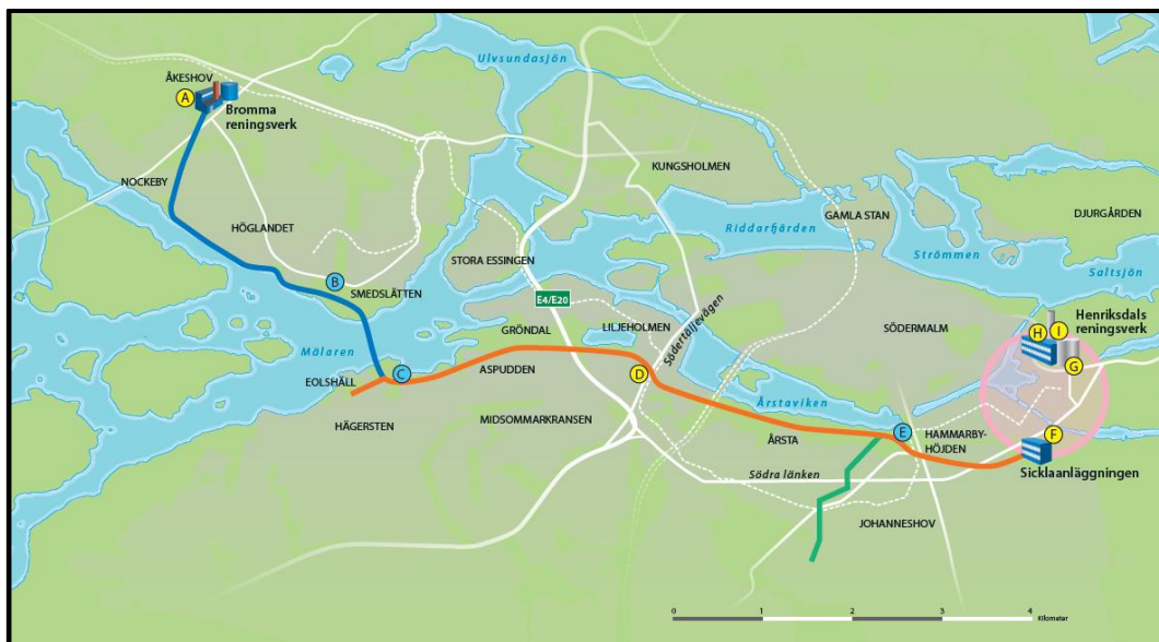
Figur 1. Tunnelsträckning. Påslag och byggarbetsplatser för tunneln är markerade med cirklar. (Källa: Stockholm Vatten)
