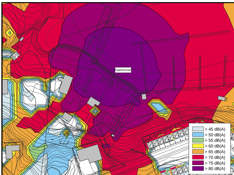
Figur 20. Arbete med topphammare för borring under anläggningsskedet. Ekvivalent ljudnivå 2 m ö mark.
